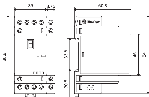
Typ 22.34 + 022.33/022.35 Schraubklemmen
