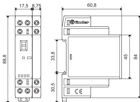
Typ 22.32 + 022.33/022.35 Schraubklemmen
