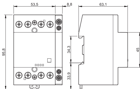
Typ 22.44/22.64 + 022.63/022.65 Schraubklemmen
