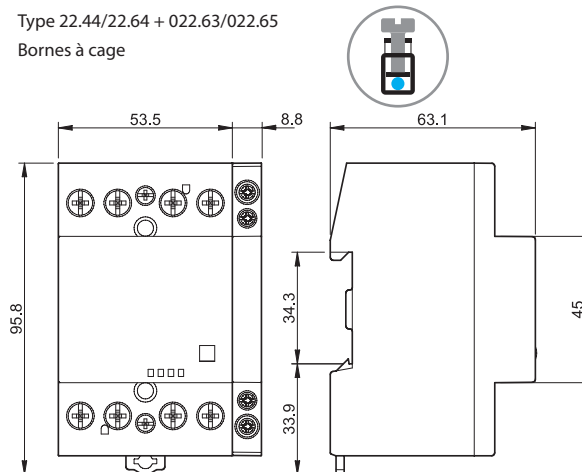
Type 022.63/022.65 Bornes à cage
