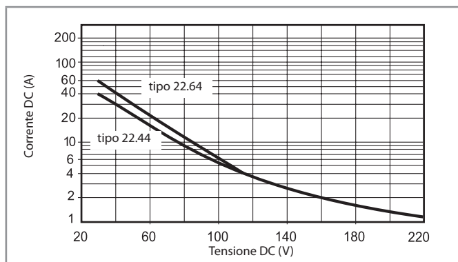
H 22 - Massimo potere di rottura su carichi in DC1 - Tipo 22.44/22.64
