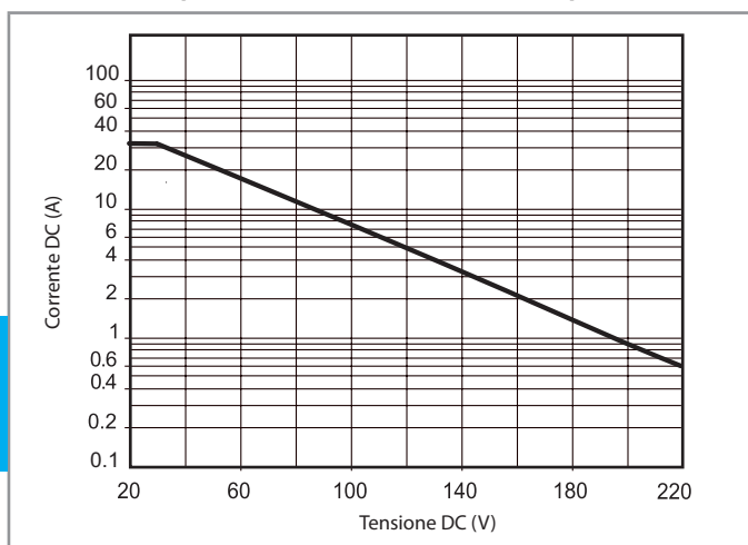
H 22 - Massimo potere di rottura su carichi in DC1 - Tipo 22.72/22.74
