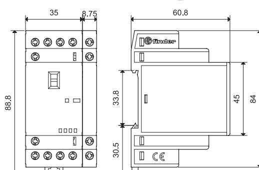
Tipi 22.34 + 022.33/022.35 Morsetti a vite
