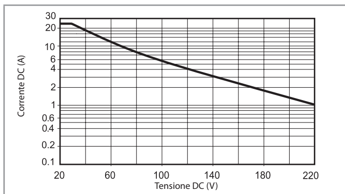
H 22 - Massimo potere di rottura su carichi in DC1 - Tipo 22.32/22.34
